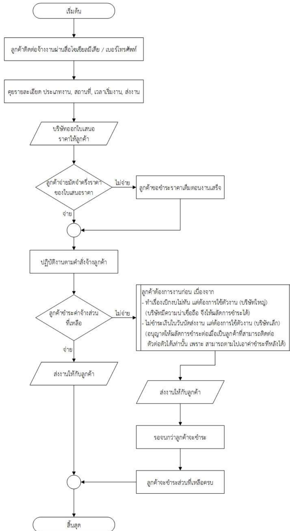
ภาพที่ 3.2 แผนผังระบบงานเดิม
